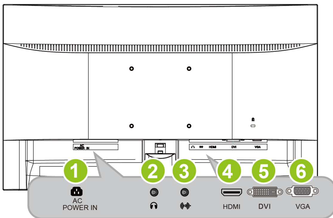
Figura 2. Conexión a un PC
